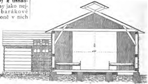
Č. 448. Baráková nemocnice.
